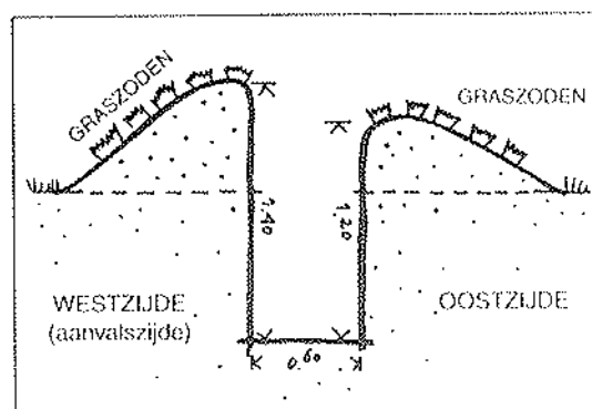
Doorsnede loopgraaf (in klei, zonder piketpalen)
